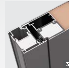
Zusätzliche Wärmedehnung im Türaufbau
